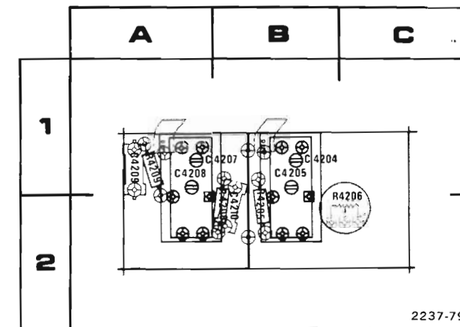
G. A4 ATTENUATOR BOARD
